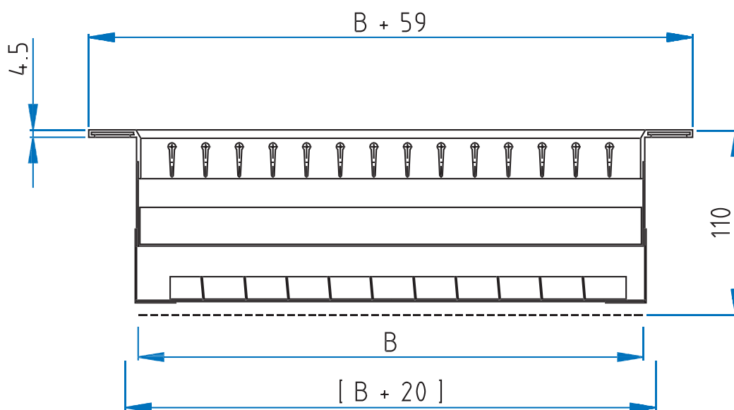
AG-540 NE AG-500 NE mit SO (Schlitzschieber)
