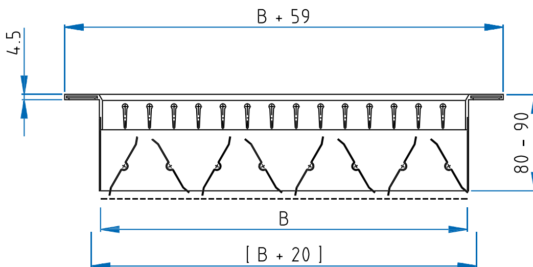
AG-630 AG-600 mit MKL-2 (gekuppelte gegenläufige Mengenregulierung)
