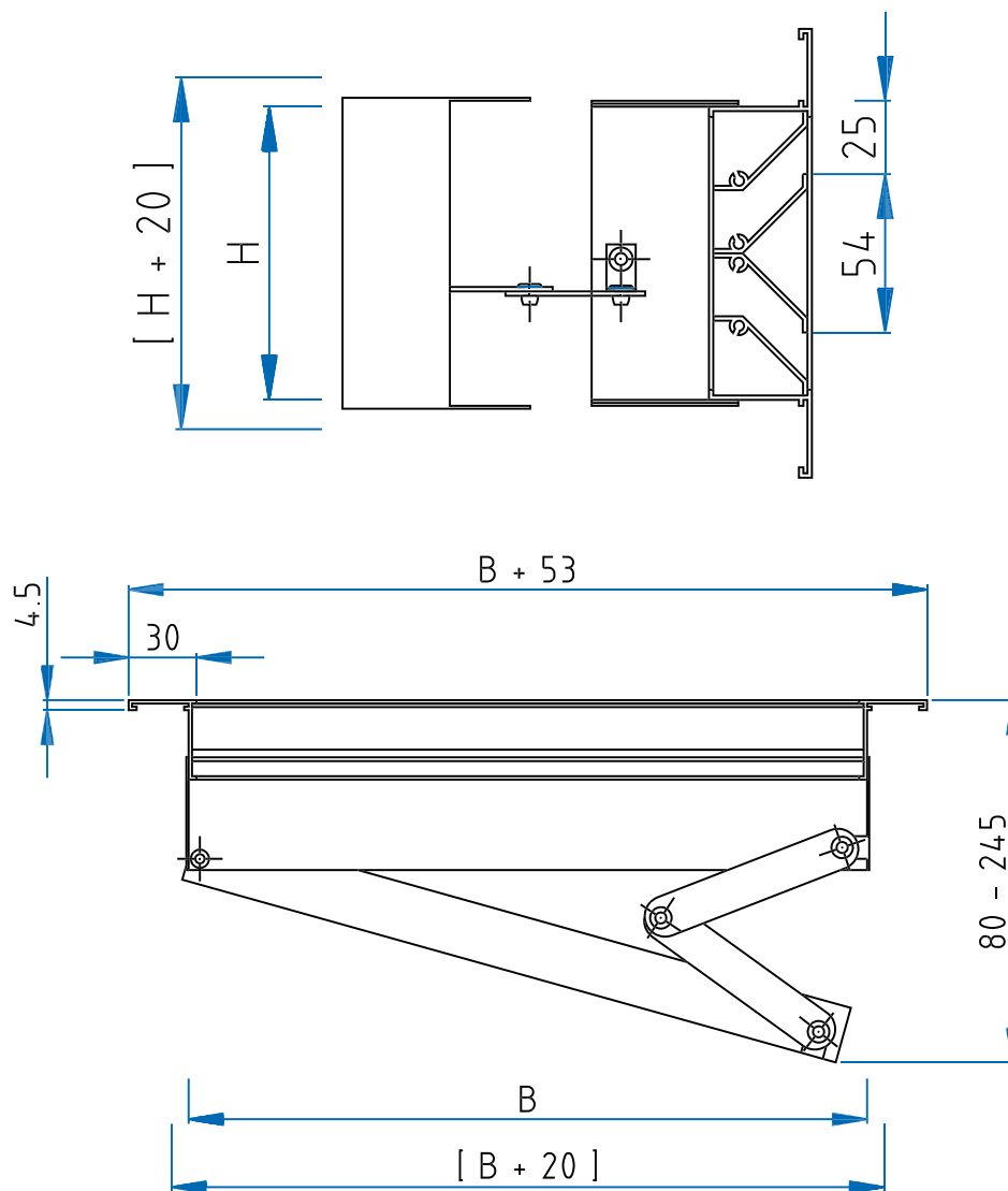
DS-110 DS-100 mit Z (einstellbare Schöpfzunge)
