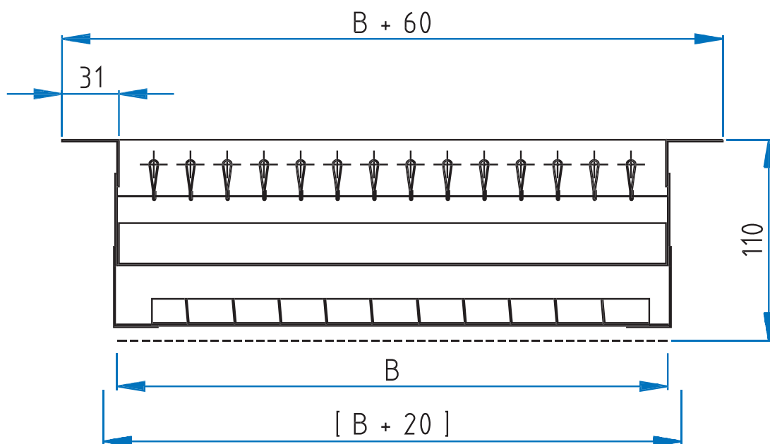
G-540 R G-500 R mit SO (Schlitzschieber)
