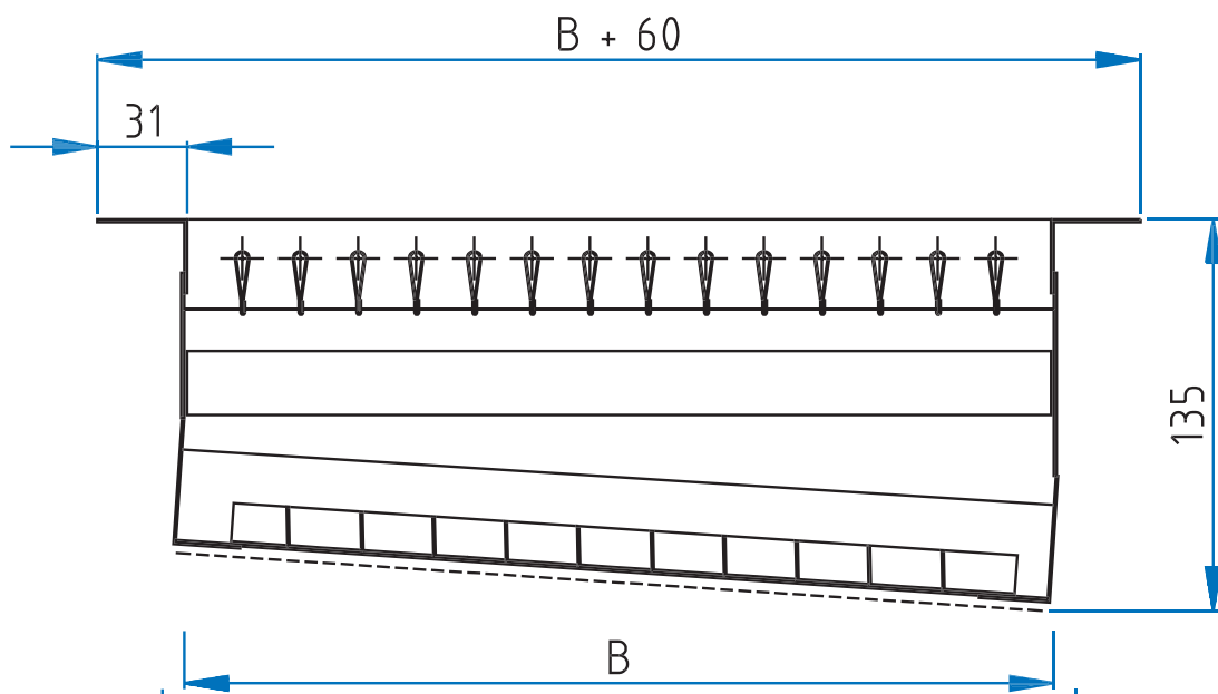
G-550 R G-500 R mit SO-A (schräger Schlitzschieber-Aufsatz)
