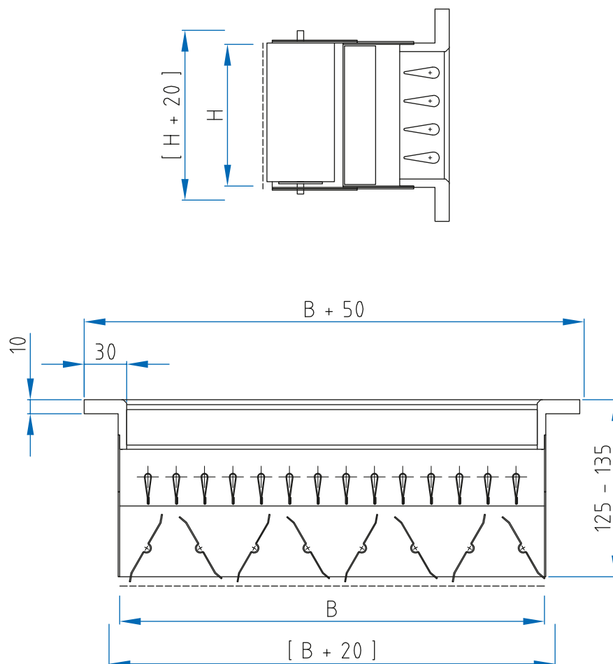
HG-230 HG-200 mit MKL-2 (gekuppelte gegenläufige Mengenregulierung)
